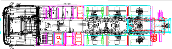
Tag-tridem WB4300
